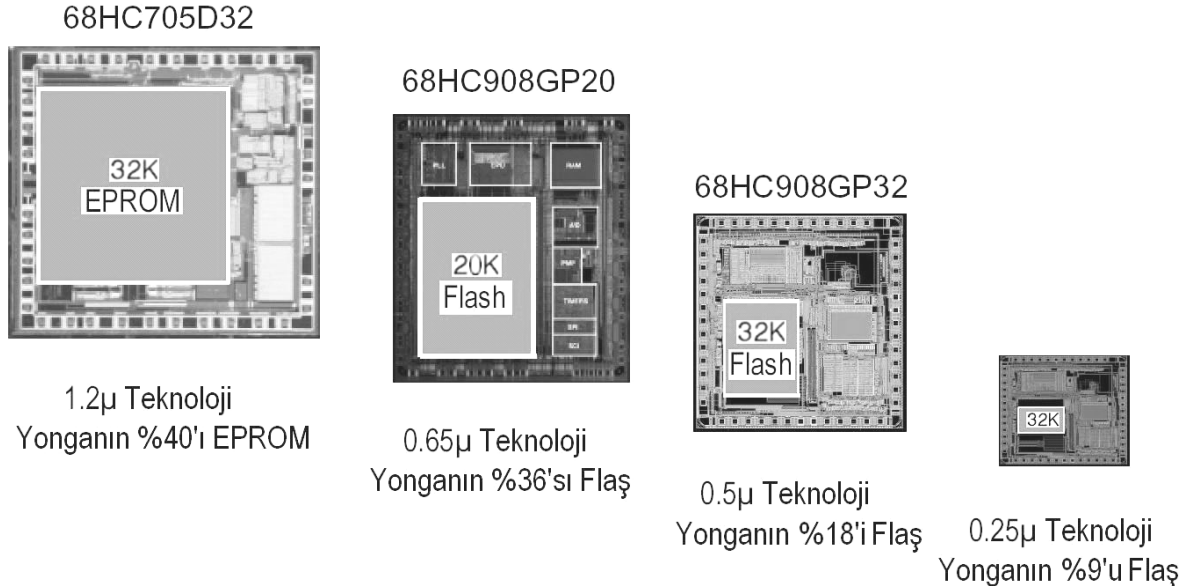
Şekil 4-5 Motorola Firmasının Mikrodenetleyici Yonga Teknolojisinin Gelişimi
